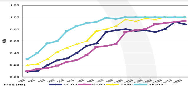
Music P - Coefficiente assorbimento acustico
