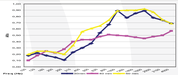
Music B - Coefficiente assorbimento acustico
